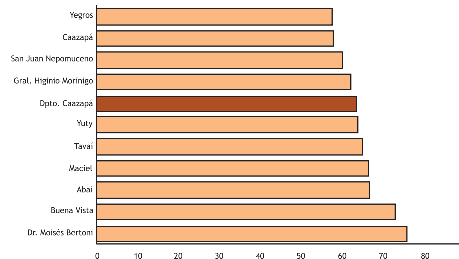
Gráfico 92. Caazapá Rural: Porcentaje de hogares con al menos una NBI por distrito, 2002.
