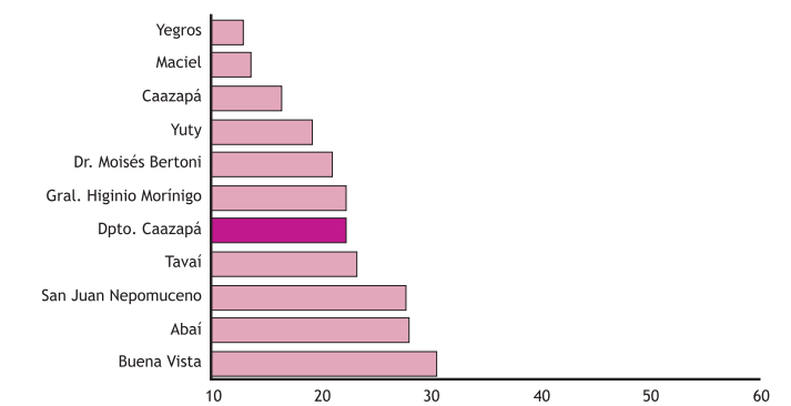
Gráfico 85. Caazapá: Porcentaje de hogares con NBI en acceso a la educación por distrito, 2002.
