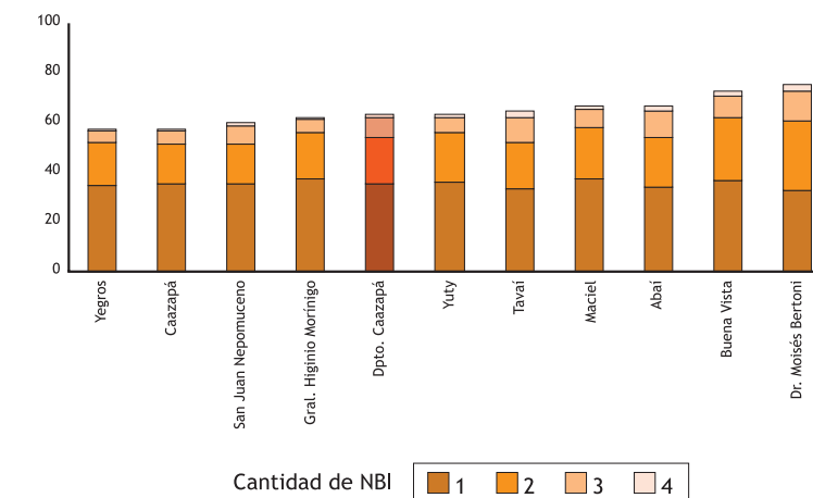
Gráfico 89. Caazapá Rural: Porcentaje de hogares por cantidad de NBI según distrito, 2002.
