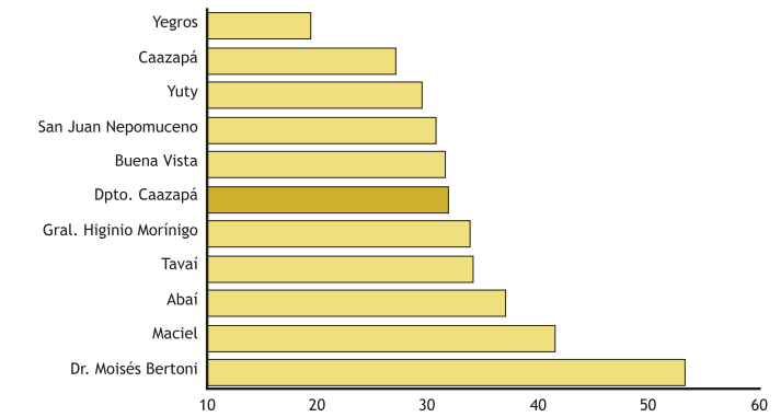
Gráfico 84. Caazapá: Porcentaje de hogares con NBI en infraestructura sanitaria por distrito, 2002.
