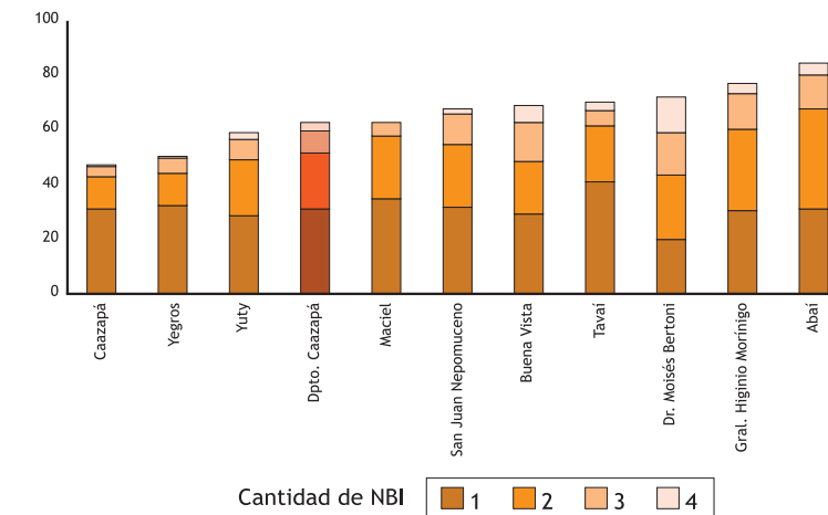
Gráfico 89. Caazapá Rural: Porcentaje de hogares por cantidad de NBI según distrito, 2002.
