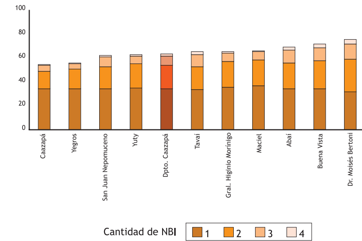
Gráfico 88. Caazapá Urbano: Porcentaje de hogares por cantidad de NBI según distrito, 2002.
