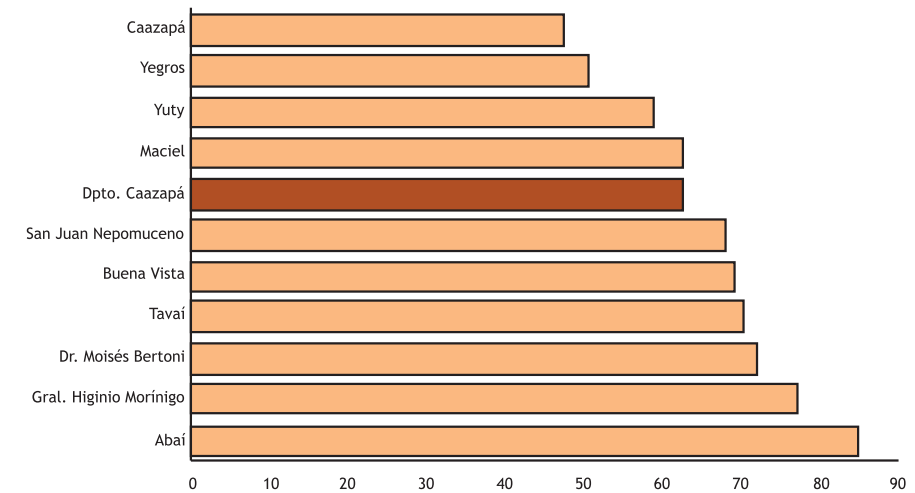
Gráfico 92. Caazapá Rural: Porcentaje de hogares con al menos una NBI por distrito, 2002.
