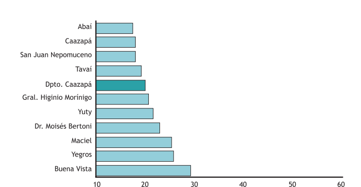
Gráfico 86. Caazapá: Porcentaje de hogares con NBI en capacidad de subsistencia por distrito, 2002.
