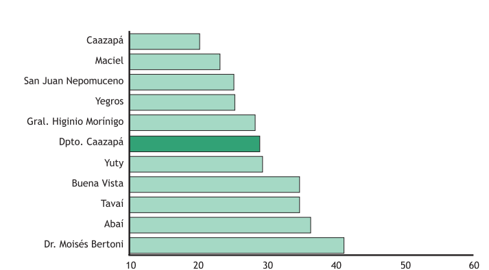
Gráfico 86. Caazapá: Porcentaje de hogares con NBI en capacidad de subsistencia por distrito, 2002.
