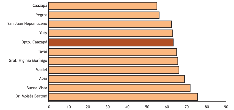
Gráfico 91. Caazapá Urbano: Porcentaje de hogares con al menos una NBI por distrito, 2002.
